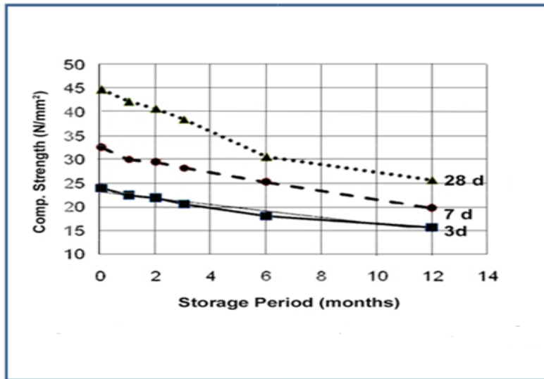
شکل (۱) کاهش مقاومت فشاری کانکریت
